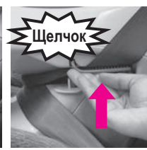
3 Нажмите на стопор ремня полностью до щелчка для надлежащей фиксации.
