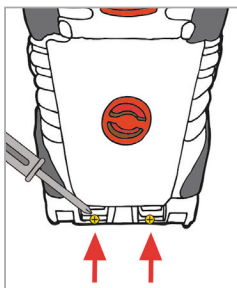
1B Нижний ремень
